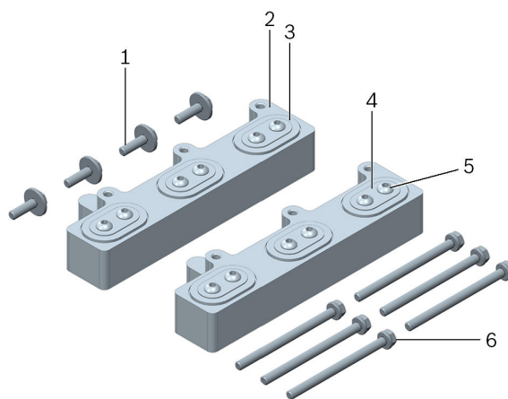
Attēls 1: Balsts T40304
