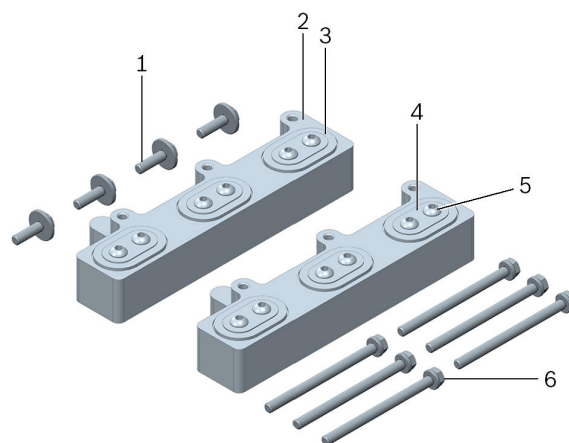
図 1: サポート T40304
