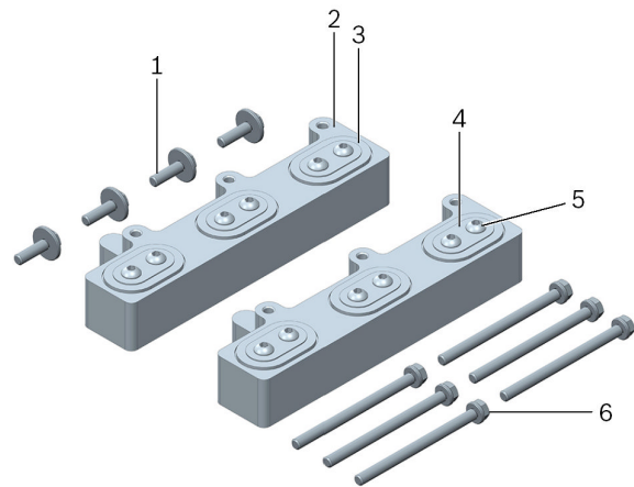
Малюнок 1: Опора T40304
