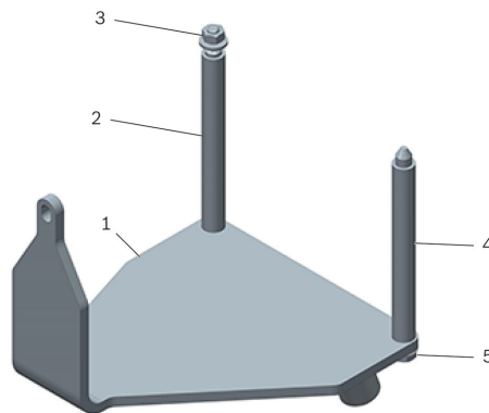
Slika 1: Držač za motor T40076
