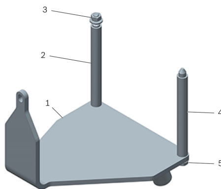
Figura 1: Supporto motore T40076
