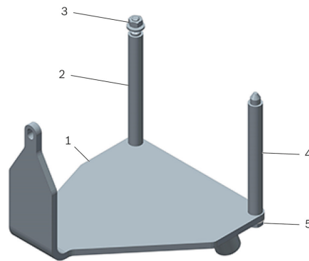
Figura 1: Soporte del motor T40076
