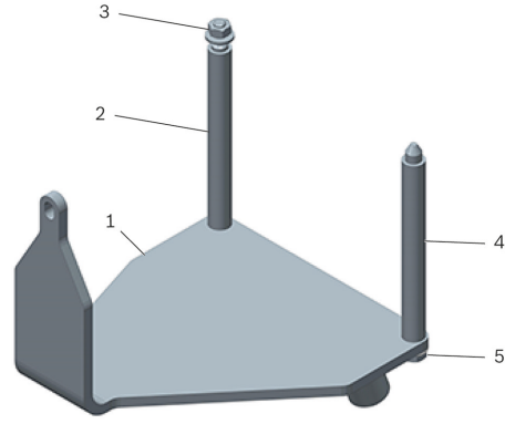
Şekil 1: Motor desteği T40076
