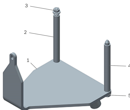
Attēls 1: Dzinēja balsts T40076
