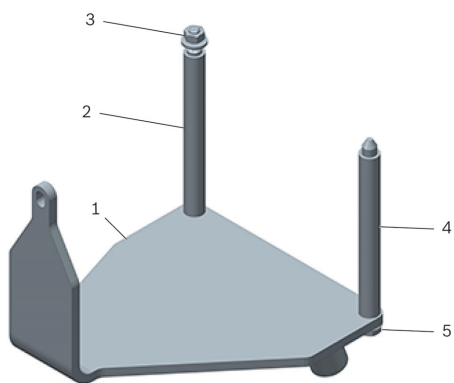
Рисунок 1: Опорное приспособление для двигателя T40076
