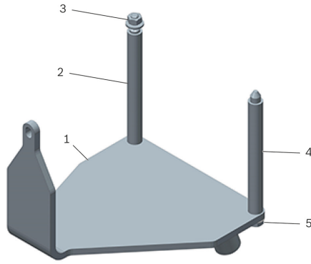
شكل 1: دعامة المحرك T40076
