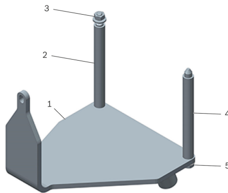
Slika 1: Opora za motor T40076
