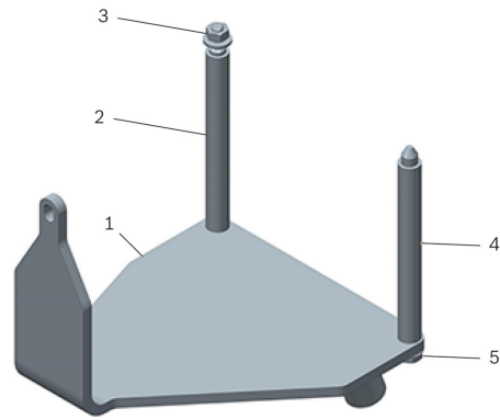
그림 1: 엔진 지지 T40076
