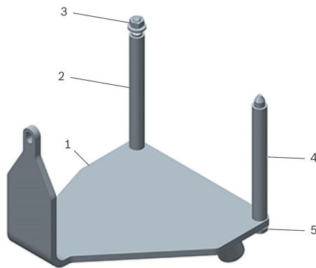
شکل 1: پایه موتور T40076
