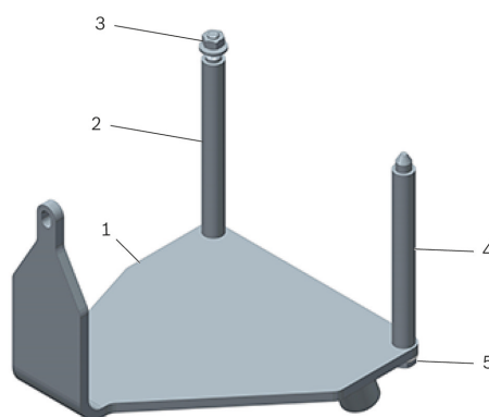
図 1: エンジンサポート T40076
