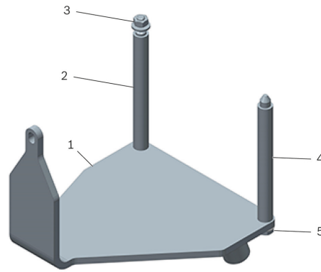
Kuva 1: Moottorikannatin T40076
