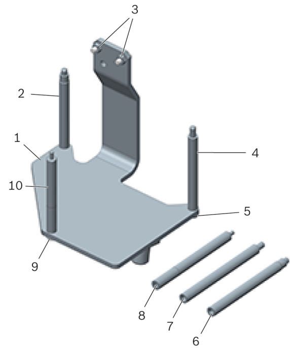
图 1: 发动机支架 T40075A
