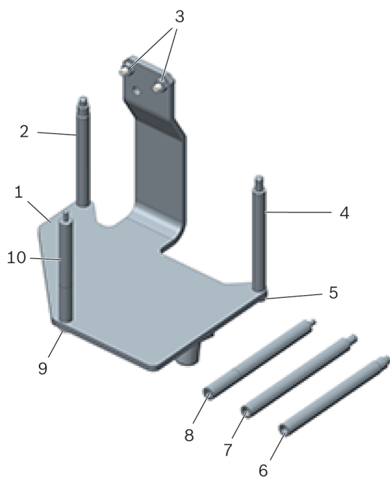
Рисунок 1: Опора для двигателя T40075A
