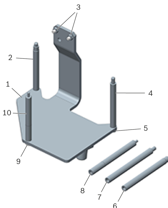
Εικόνα 1: Στήριγμα κινητήρα T40075A
