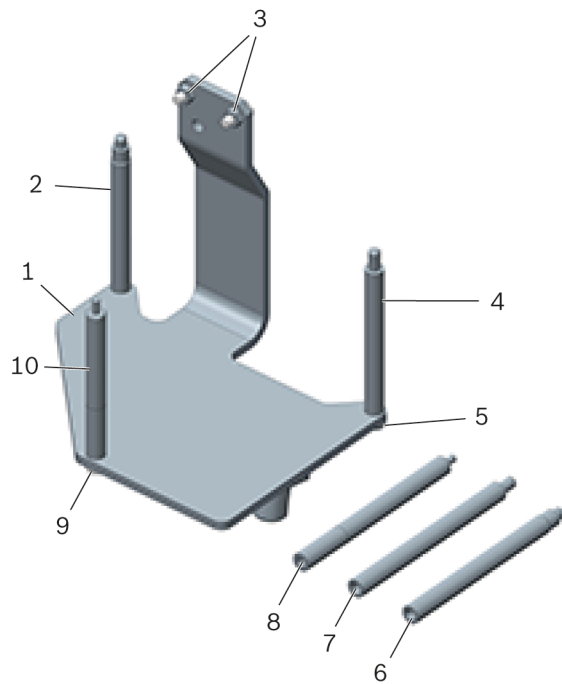
איור 1: תושבת מנוע T40075A
