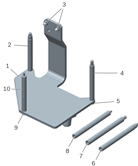
Малюнок Опора для двигуна T40075A 1:
