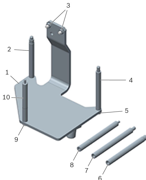
Imagen 1: Soporte del motor T40075A
