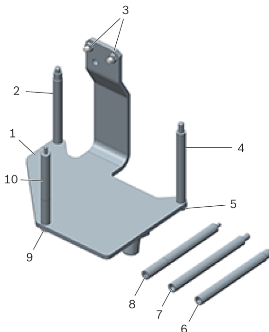
Obrázek 1: Podpěra motoru T40075A
