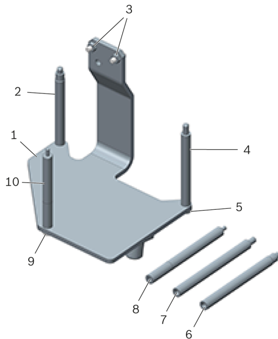
شکل 1: پایه موتور T40075A
