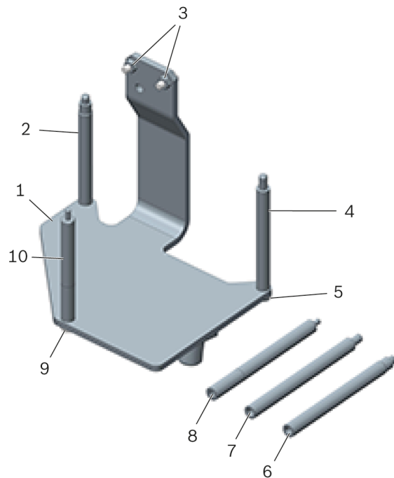
Figură 1: Suport de motor T40075A
