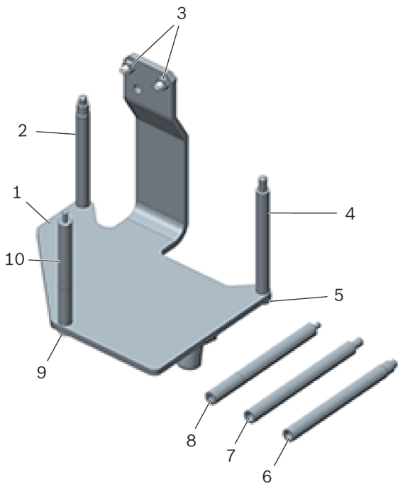
Figura 1: Soporte del motor T40075A
