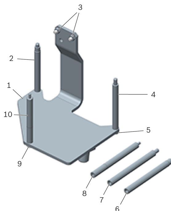
図 1: エンジンサポート T40075A
