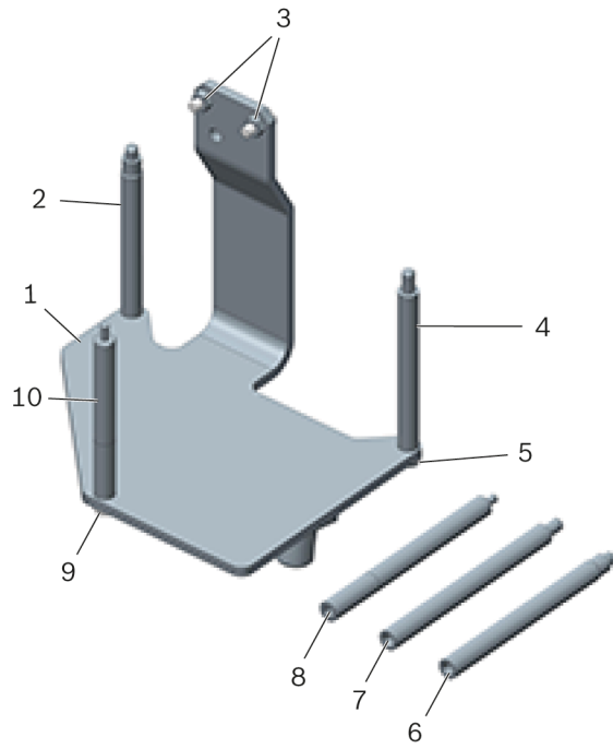
شكل 1: دعامة المحرك T40075A
