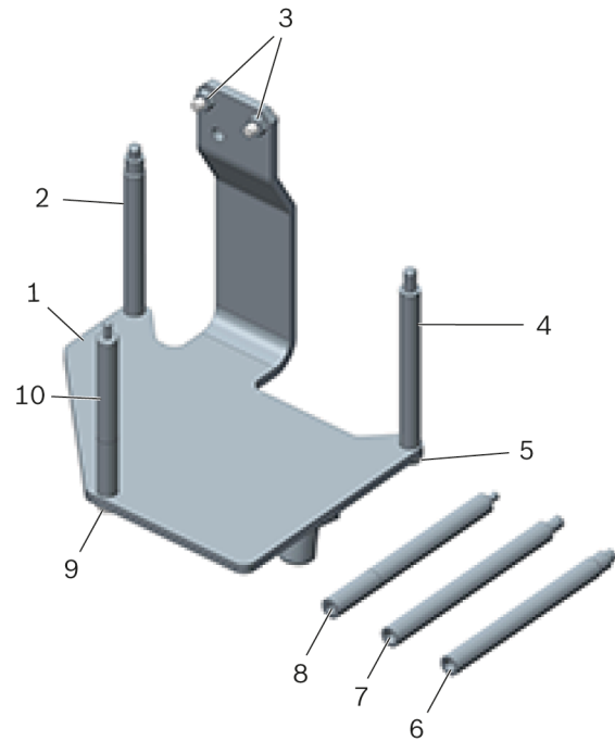
그림 1: 엔진 지지 T40075A
