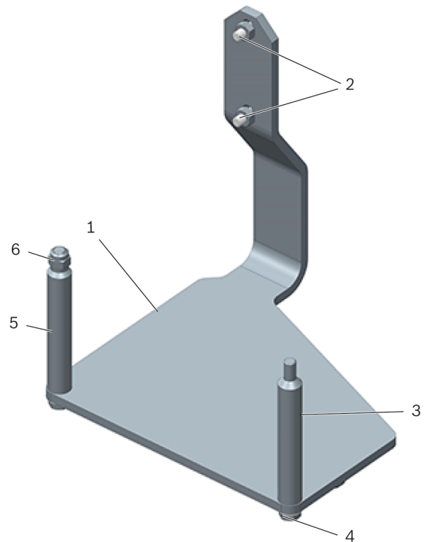
Малюнок Опора для двигуна T40074 1:
