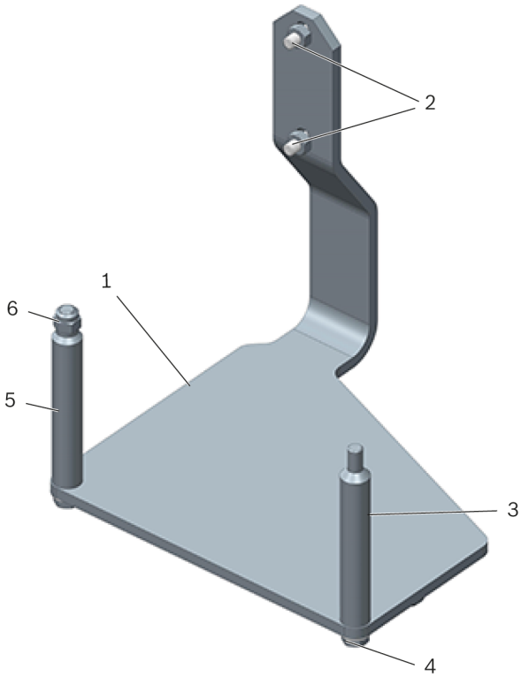
图 1: 发动机支架 T40074
