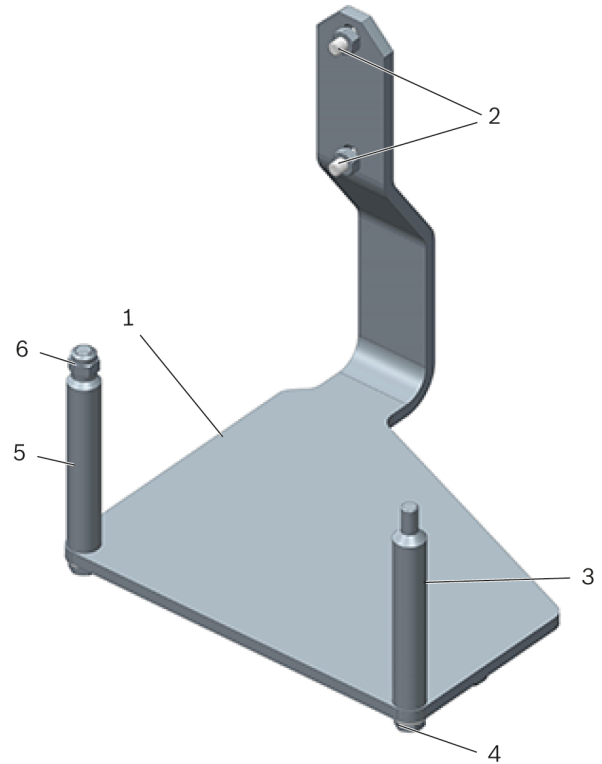
Kuva 1: Moottorikannatin T40074
