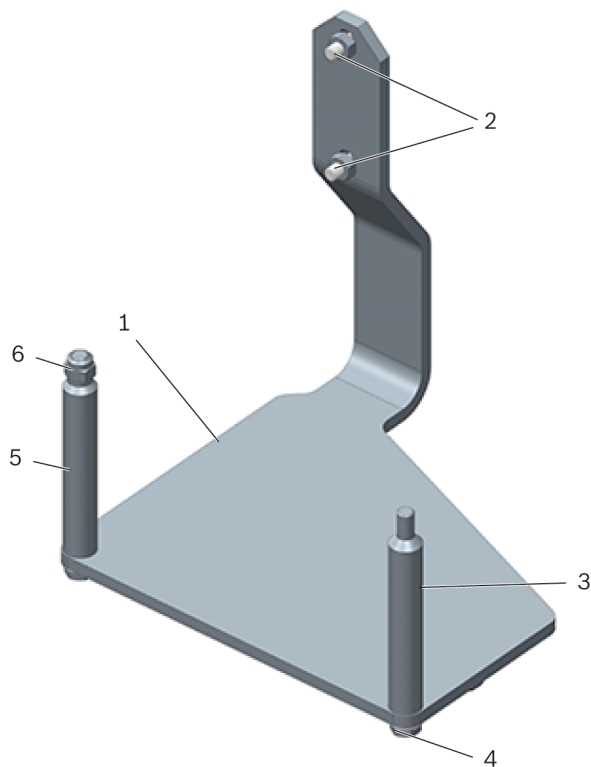
圖 1: 引擎支撐架 T40074
