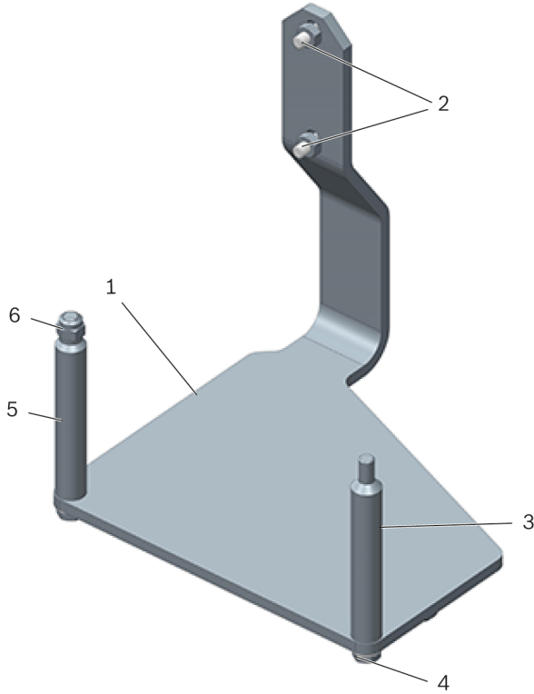
شكل 1: دعامة المحرك T40074
