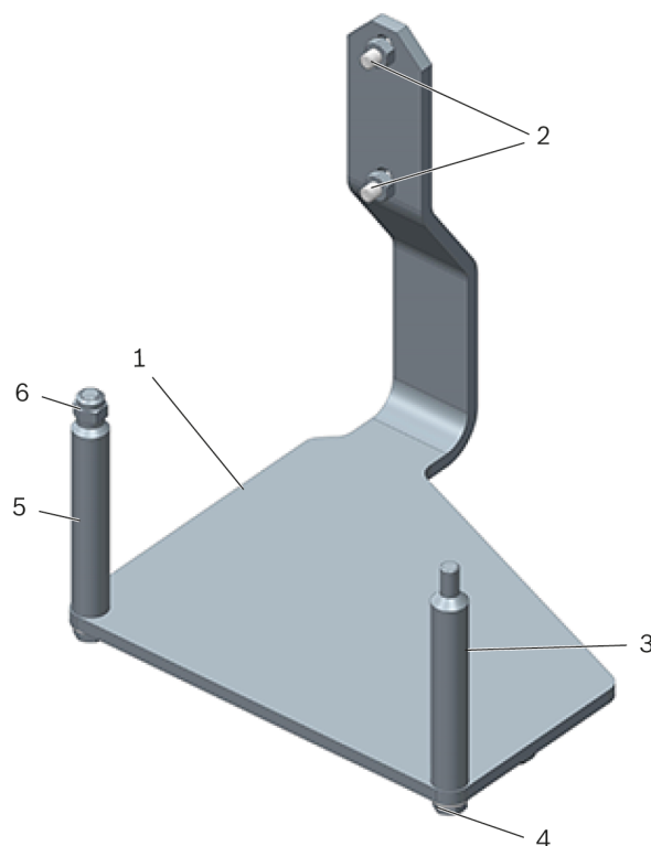
Figure 1: Support de moteur T40074
