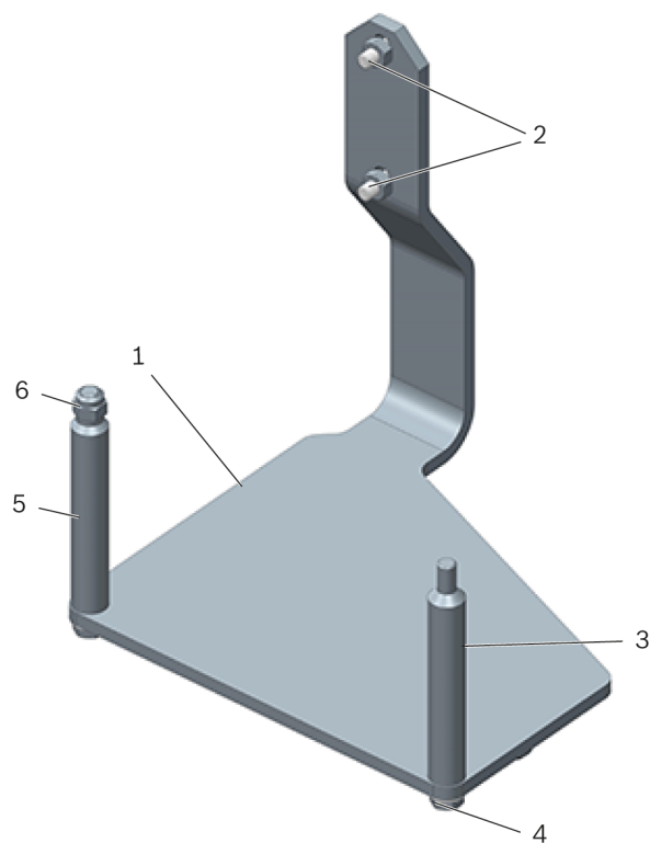
Figură 1: Suport de motor T40074
