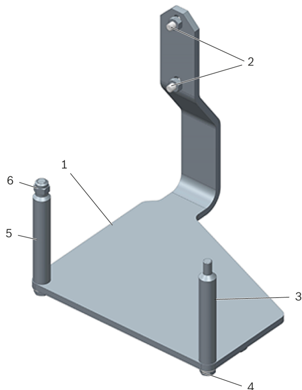
Imagen 1: Soporte del motor T40074
