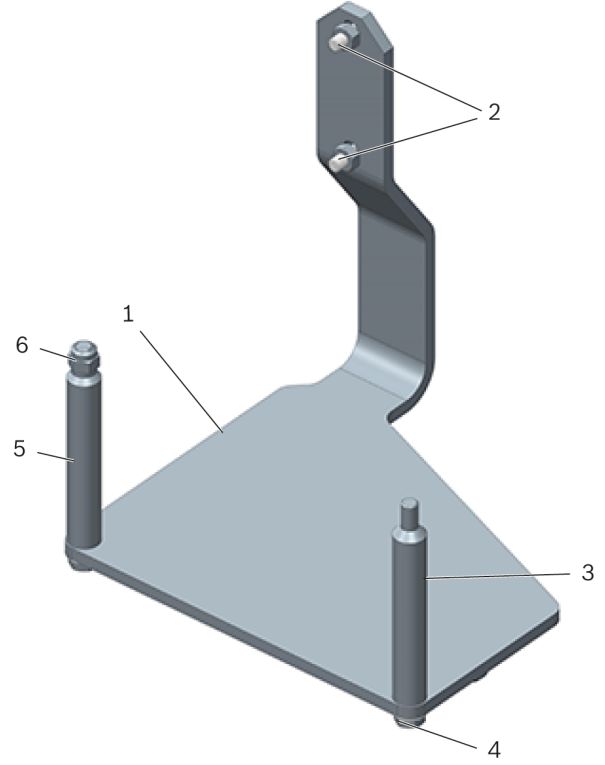
Şekil 1: Motor desteği T40074
