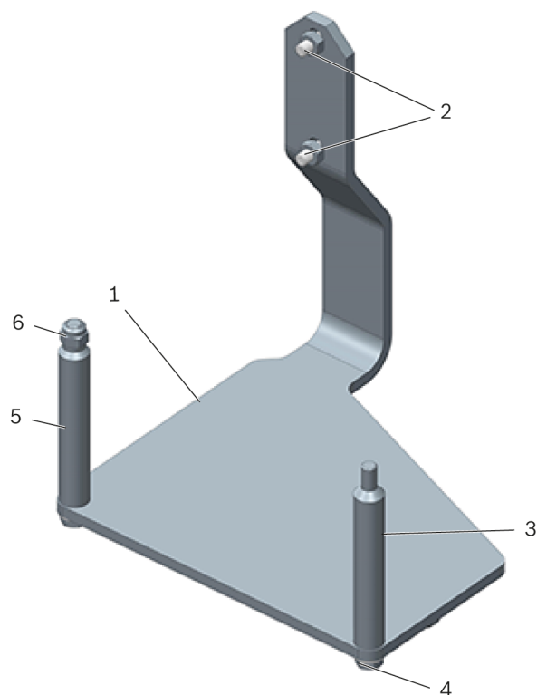
Attēls 1: Dzinēja balsts T40074
