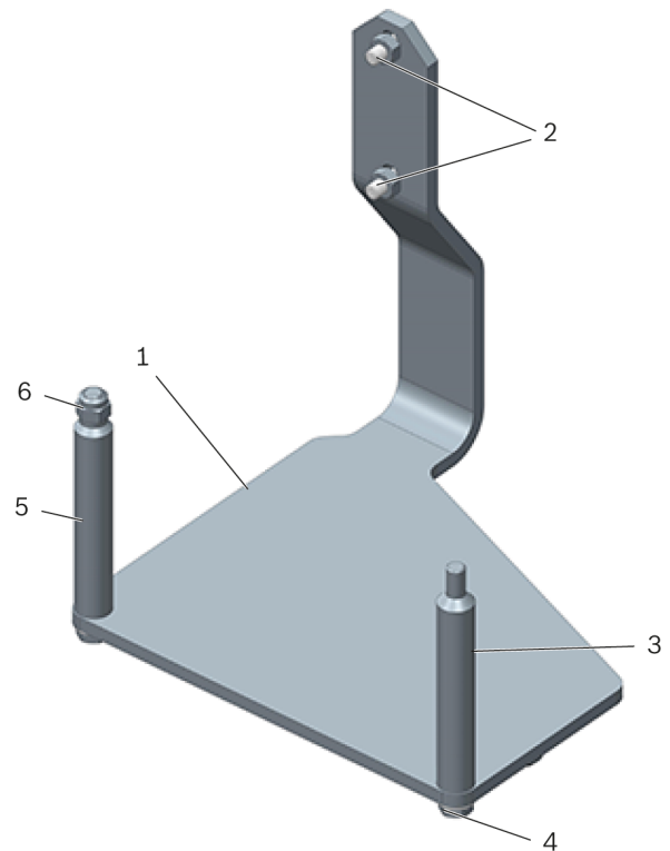
Рисунок 1: Опора для двигателя T40074
