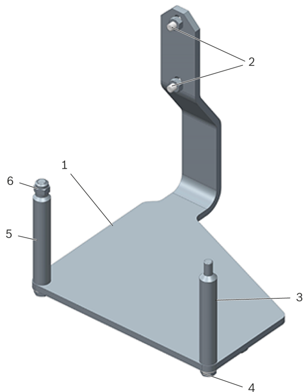
Фигура 1: Опора на двигател T40074
