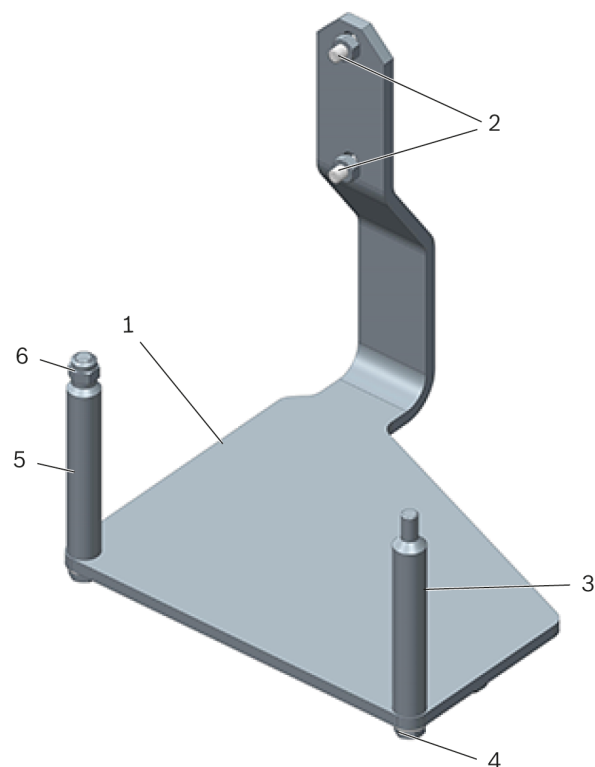
図 1: エンジンサポート T40074
