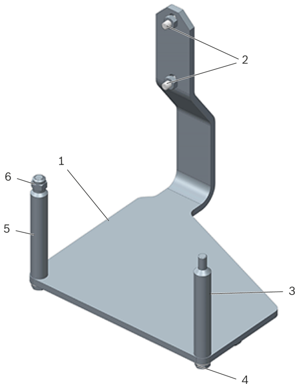
איור 1: תושבת מנוע T40074
