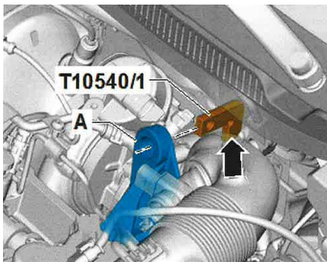
Fig. 2: Inserirre l'adattatore T10540/1
