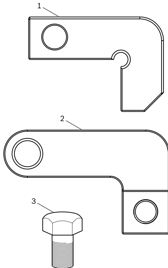
Fig. 1: Adattatore T10540
