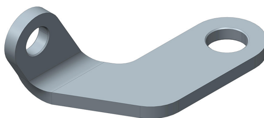
圖 1: 托架 T10358
