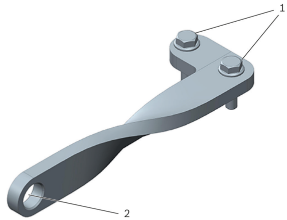
Малюнок Консоль T10339
