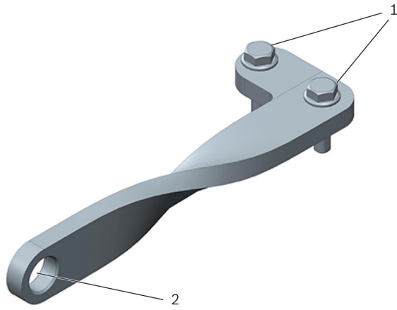
شكل 1: كتيفة T10339
