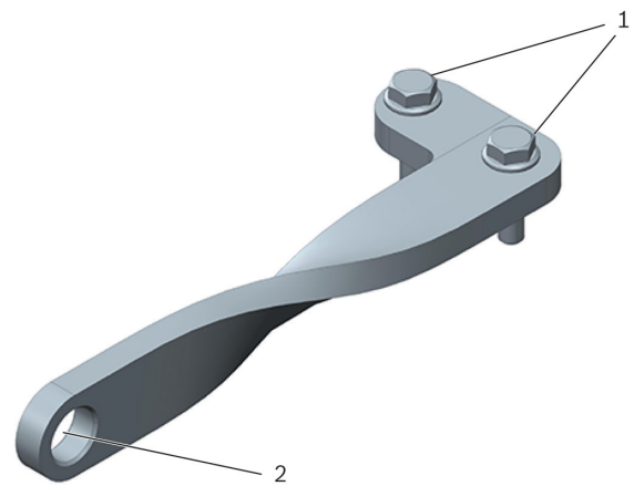
Рисунок 1: Кронштейн T10339
