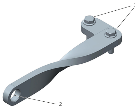
Imagen 1: Soporte angular T10339
