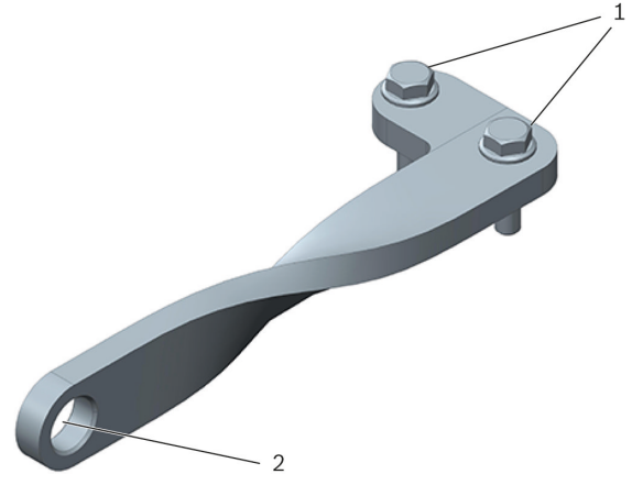
Şekil 1: T10339 Braket
