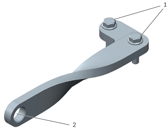
Слика Држач T10339
