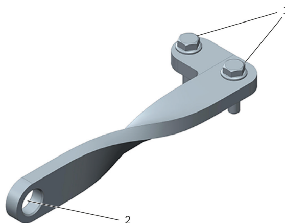
Rysunek 1: Wspornik T10339
