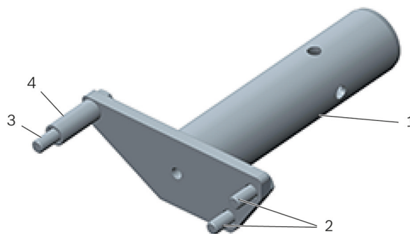
Imagen 1: Soporte de la caja de engranajes T10316
