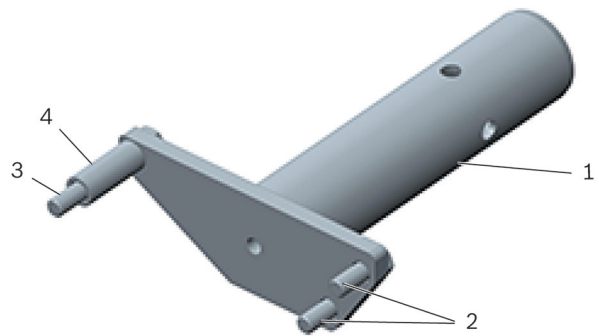
Рисунок 1: Опорное приспособление для коробки передач T10316
