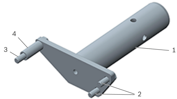
그림 1: 기어박스 지지 T10316
