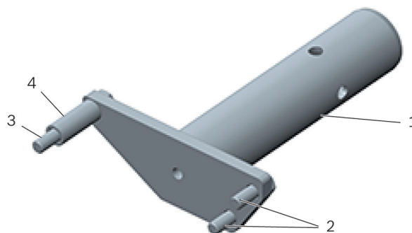
Joonis 1: Käigukastitugi T10316
