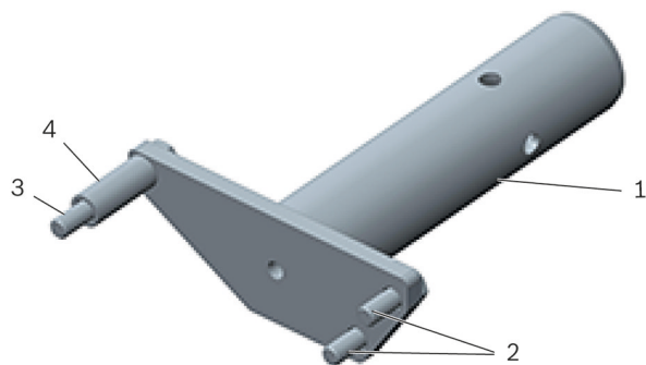
איור 1: תושבת תיבת תמסורת T10316
