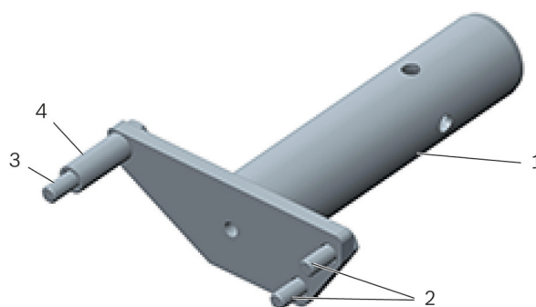
Obrázok 1: Podpera prevodovky T10316
