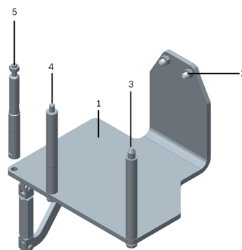
圖 1: 引擎支撐架 T10229A
