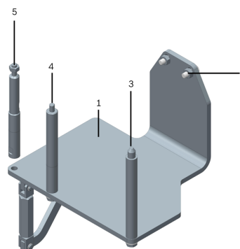
Obrázek 1: Podpěra motoru T10229A
