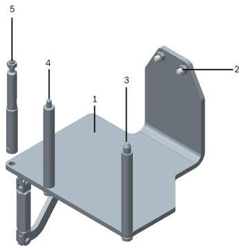
شکل 1: پایه موتور T10229A
