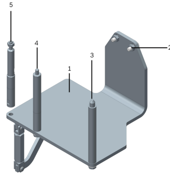
그림 1: 엔진 지지 T10229A
