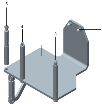
Figură 1: Suportul de motor T10229A
