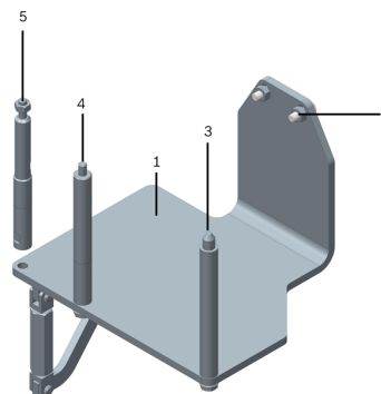
Слика 1: Потпора за моторот T10229A
