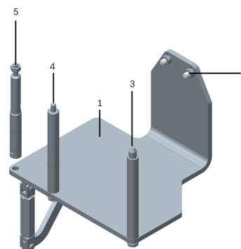
図 1: エンジンサポート T10229A
