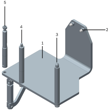
شكل 1: دعامة المحرك T10229A
