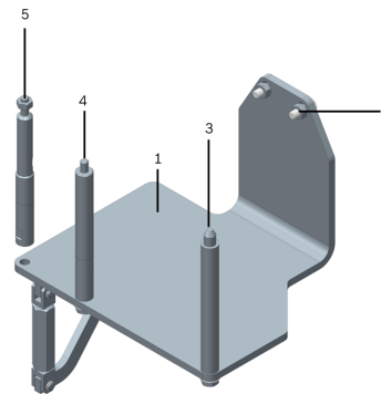
Slika 1: Držač za motor T10229A
