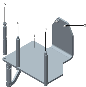
Рисунок 1: Опорное приспособление для двигателя T10229A
