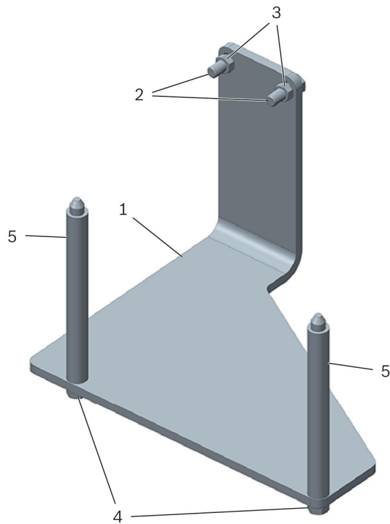
شکل 1: پایه موتور T10224
