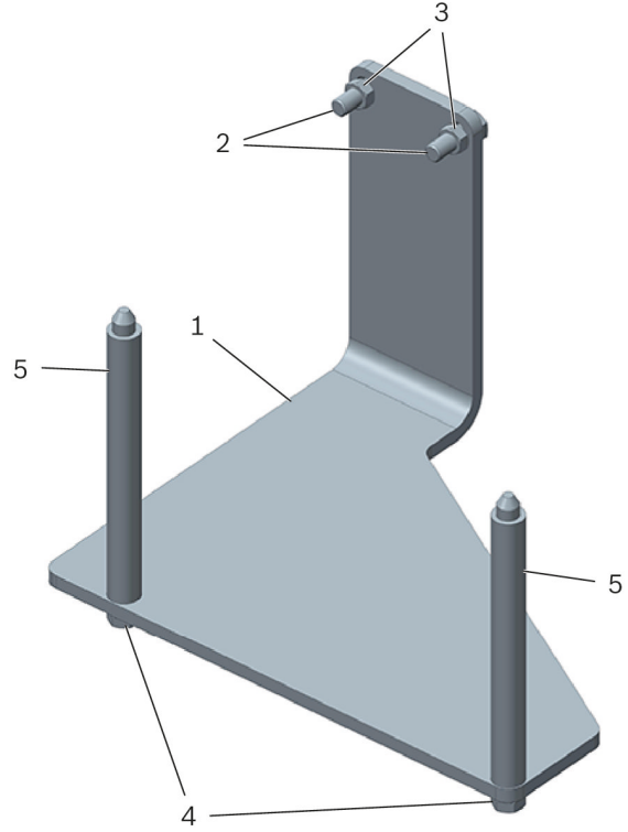
Şekil 1: Motor desteği T10224
