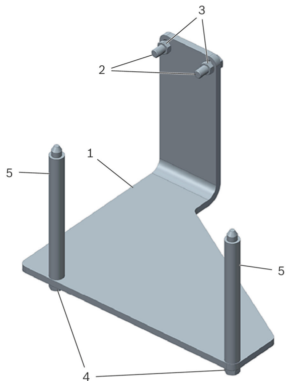
Рисунок 1: Опора для двигателя T10224
