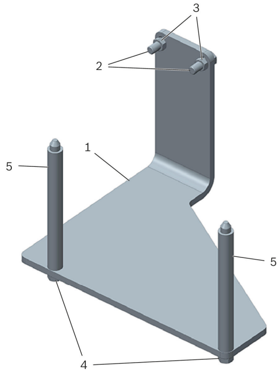
그림 1: 엔진 지지 T10224
