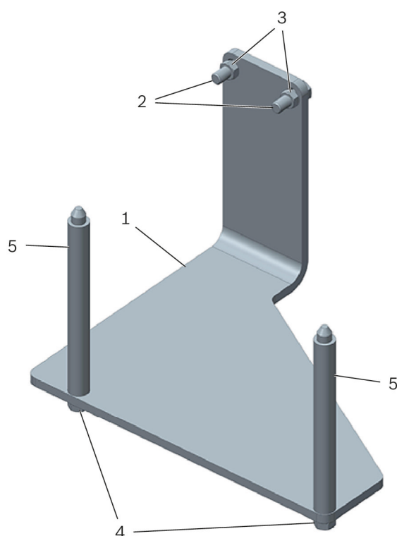
圖 1: 引擎支撐架 T10224
