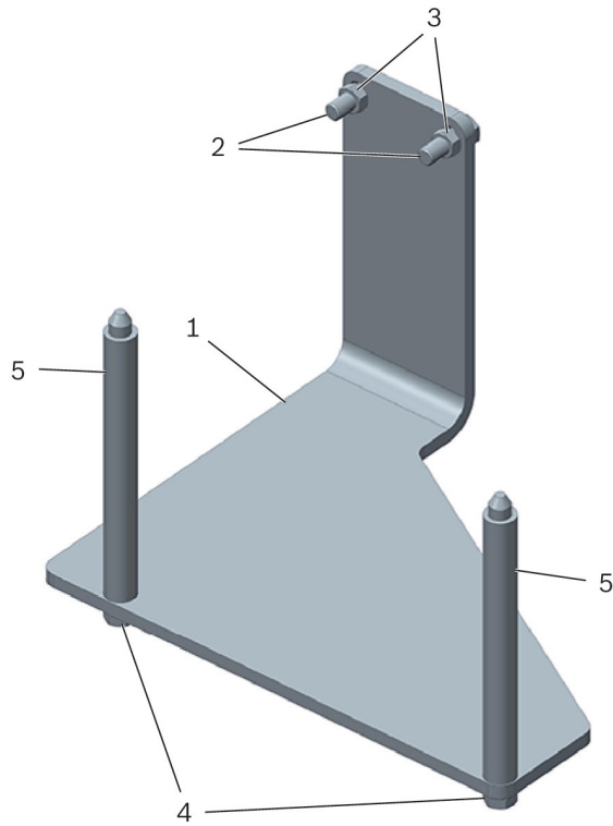
شكل 1: دعامة المحرك T10224
