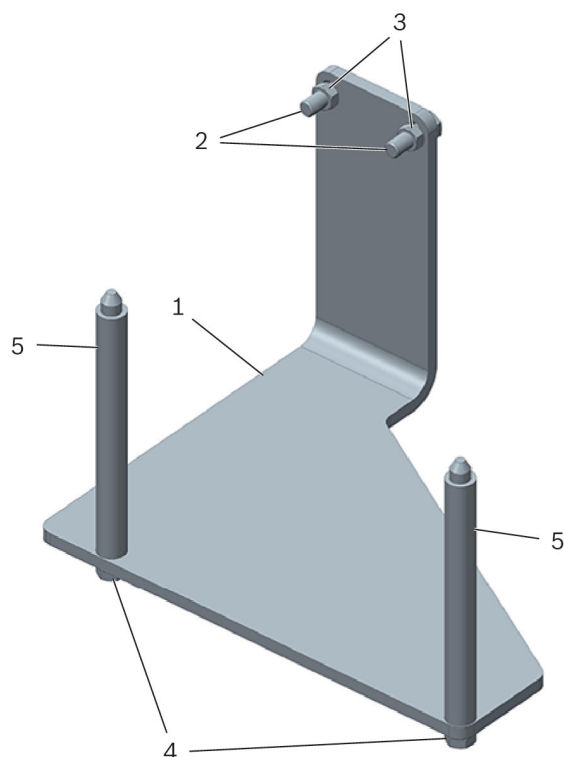
Joonis 1: Mootori tõstetala T10224
