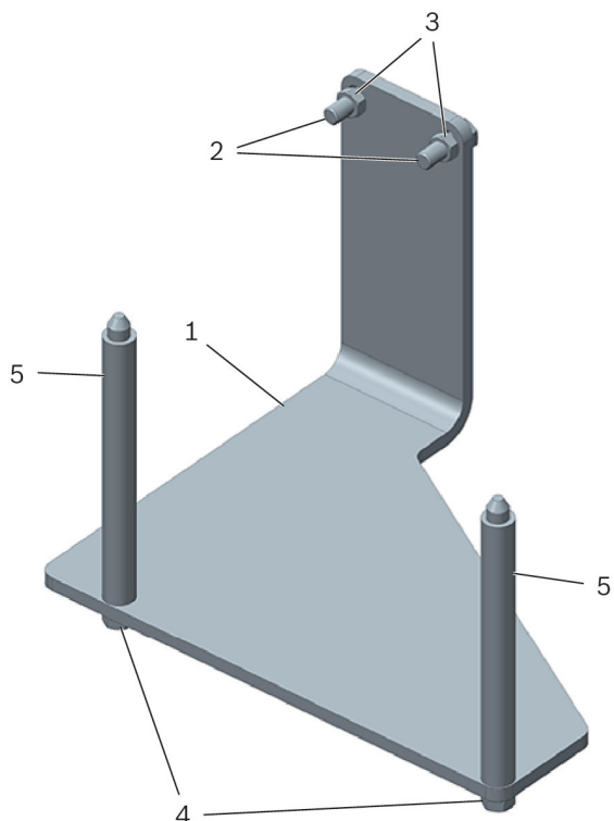
Фигура 1: Опора на двигател T10224
