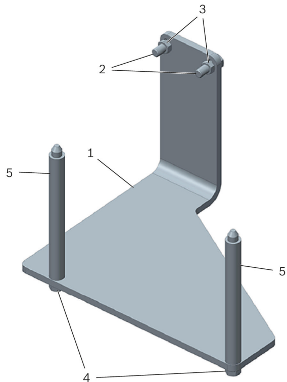
Малюнок Опора для двигуна T10224
