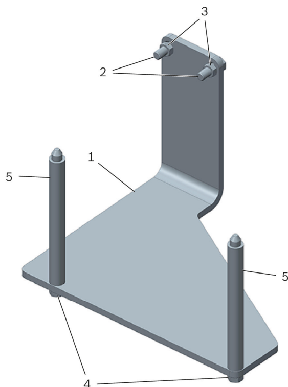
Figură 1: Suport de motor T10224
