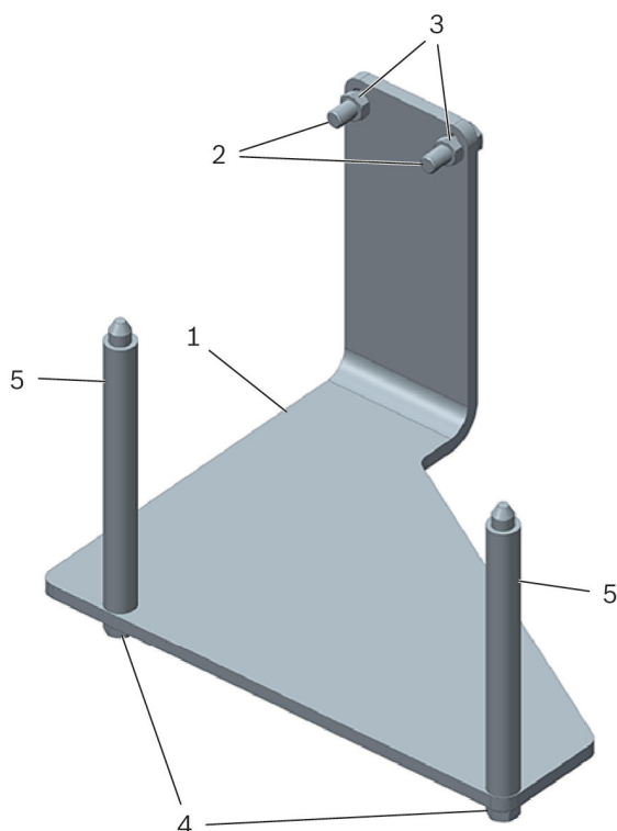
图 1: 发动机支架 T10224
