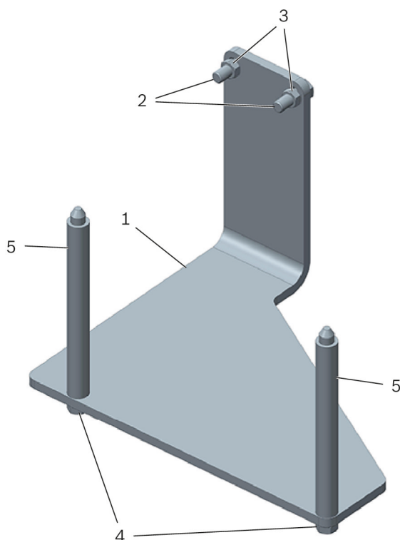
Attēls 1: Dzinēja balsts T10224
