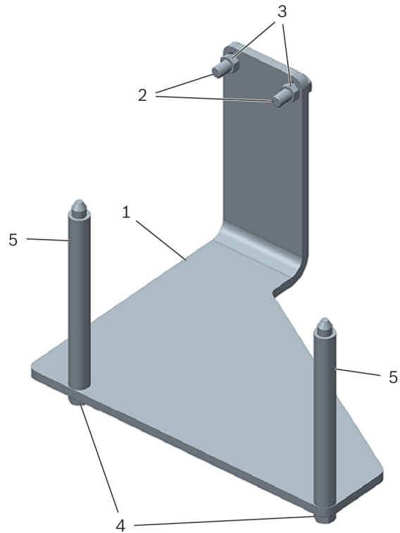
Kuva 1: Moottorikannatin T10224
