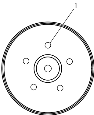
Fig. 2: Posizione del foro del bullone della ruota
