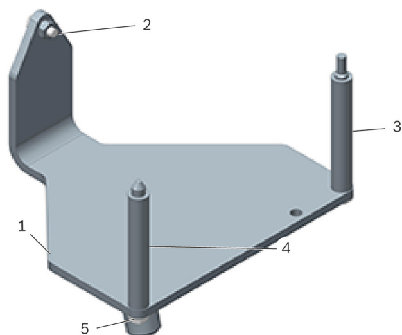
Figure 1: Support de moteur T10012
