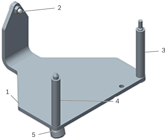
شكل 1: دعامة المحرك T10012
