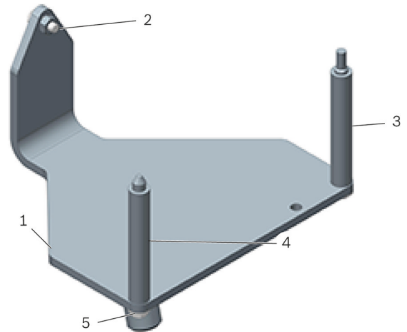
그림 1: 엔진 지지 T10012
