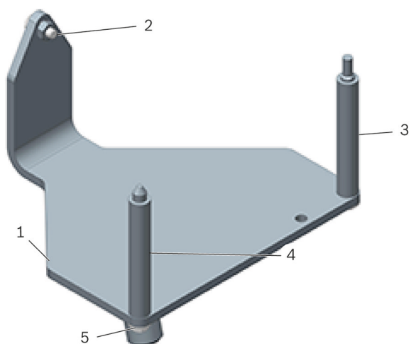
Рисунок 1: Опора для двигателя T10012
