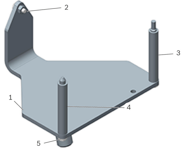
Şekil 1: Motor desteği T10012
