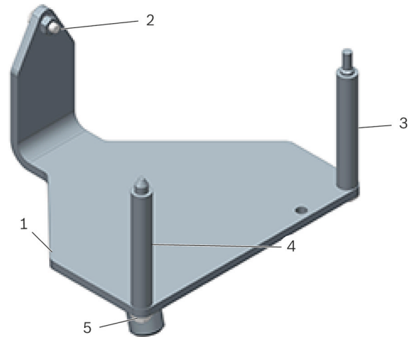
Kuva 1: Moottorikannatin T10012
