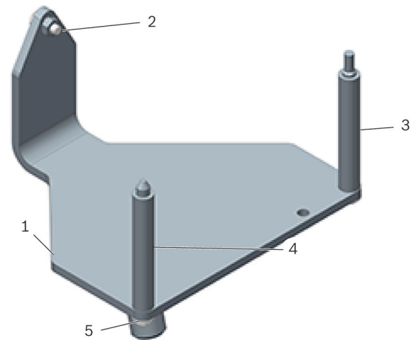
图 1: 发动机支架 T10012
