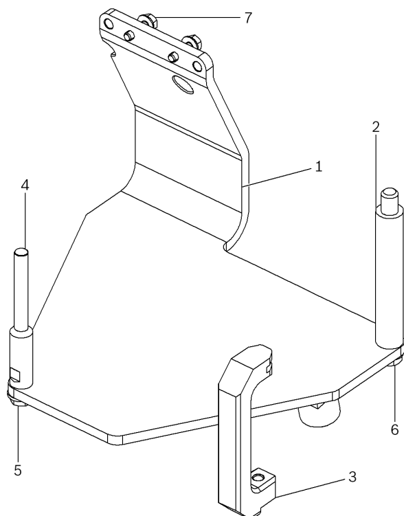
Εικόνα 1: Στήριγμα κινητήρα T03000A
