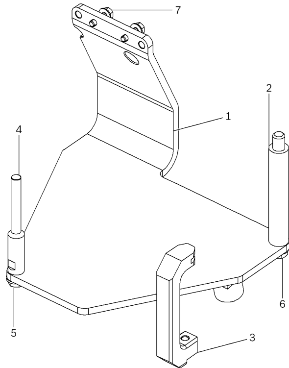
Kuva 1: Moottorikannatin T03000A
