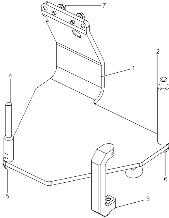
شكل 1: دعامة المحرك T03000A
