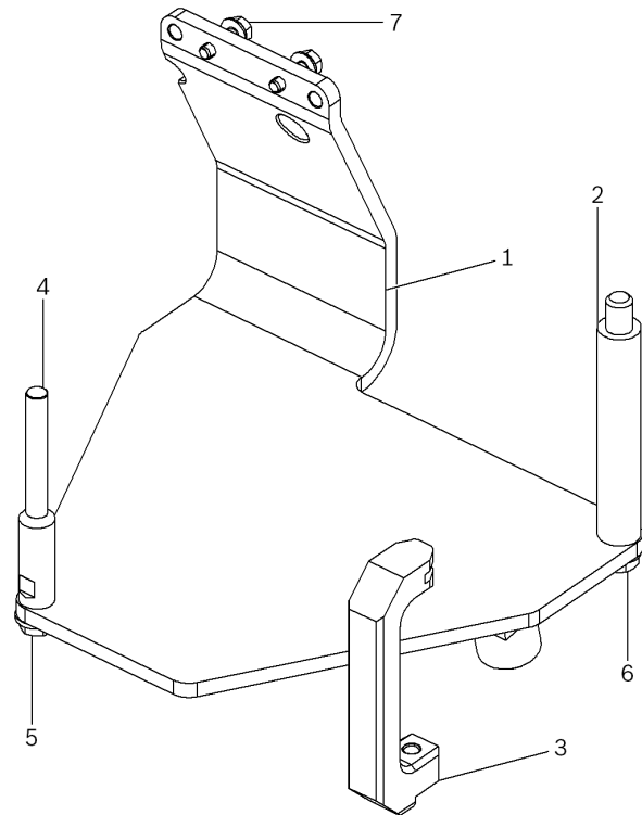
그림 1: 엔진 지지 T03000A
