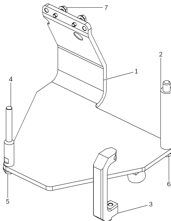
Рисунок 1: Опорное приспособление для двигателя T03000A
