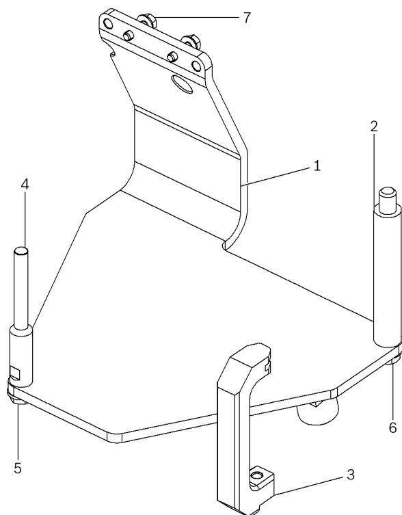
Joonis 1: Mootori tõstetala T03000A
