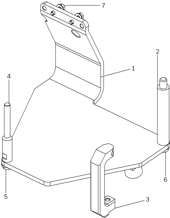
图 1: 发动机支架 T03000A
