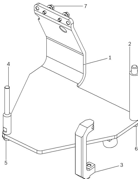
Attēls 1: Dzinēja balsts T03000A
