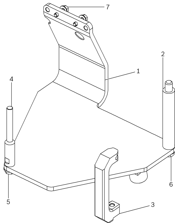
Малюнок 1: Опора для двигуна T03000A
