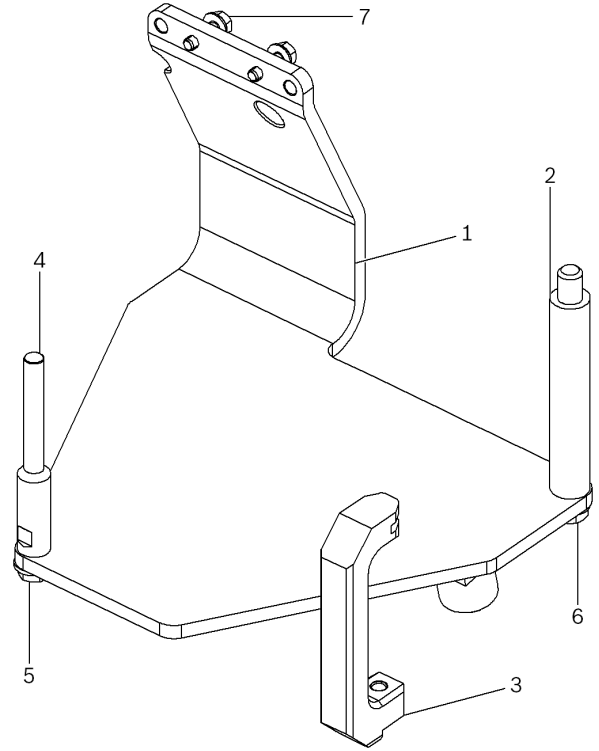
Şekil 1: Motor desteği T03000A
