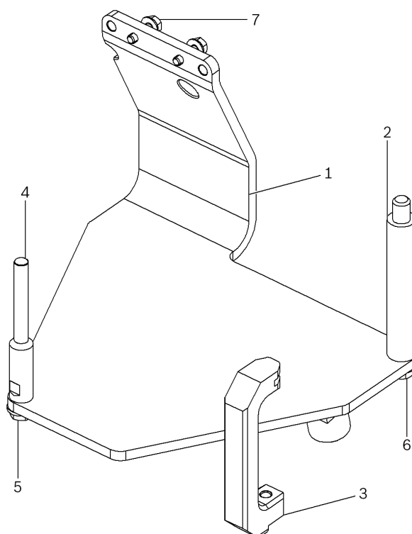
Ábra 1: T03000A motortartó
