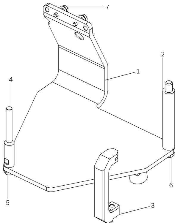
Imagen 1: Soporte del motor T03000A
