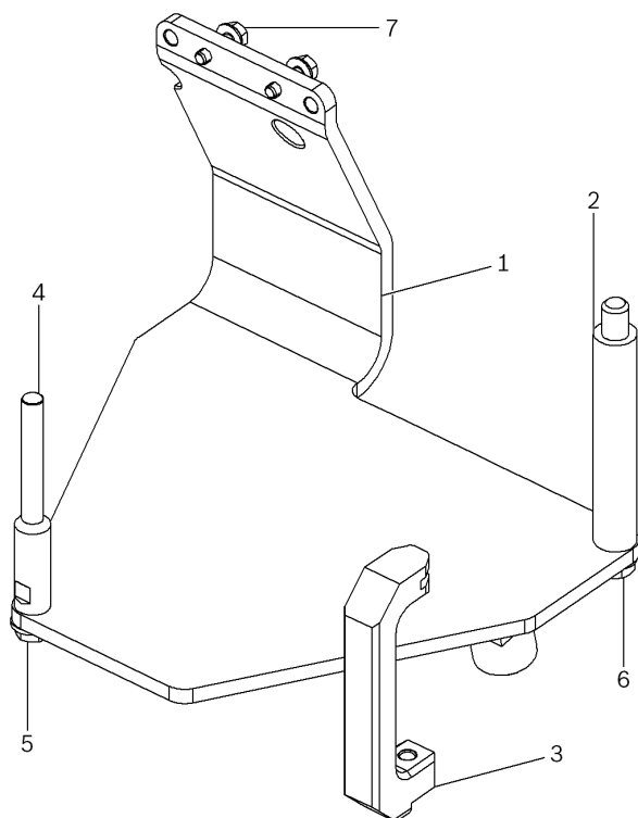
شکل 1: پایه موتور T03000A
