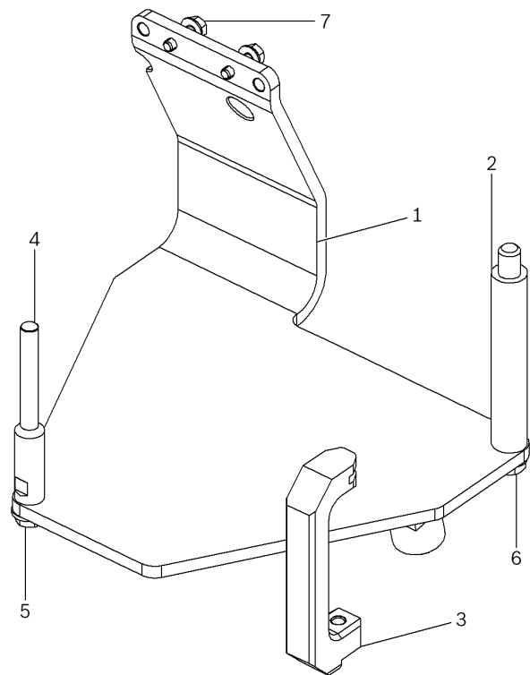
圖 1: 引擎支撐架 T03000A
