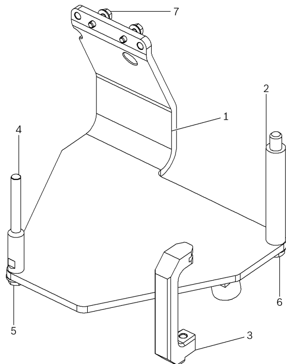
Afbeelding 1: Motorstøtte T03000A
