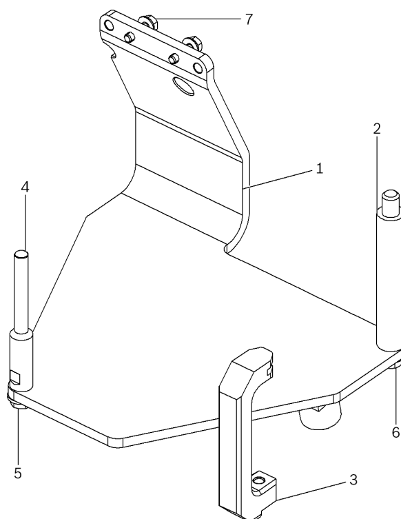
Rysunek 1: Wspornik silnika T03000A
