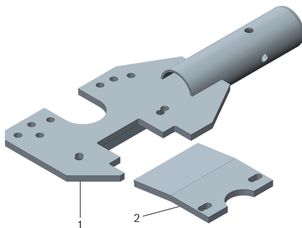
Figura 1: Soporte de la caja de cambios 3221B
