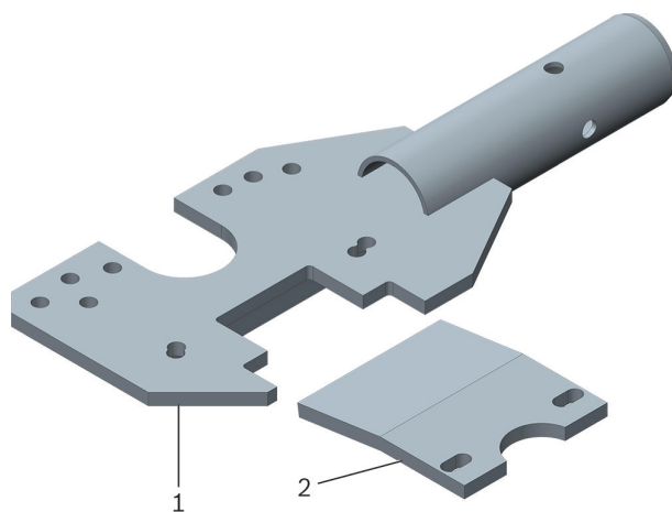
Figura 1: Suporte de caixa de transmissão 3221B
