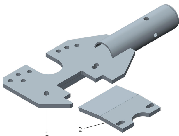
Рисунок 1: Опорное приспособление для коробки передач 3221B
