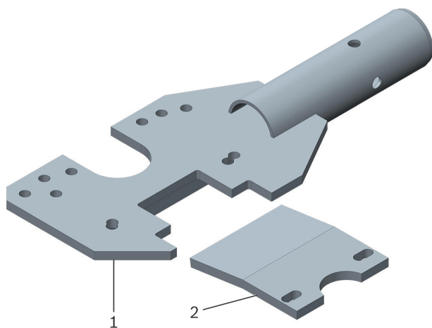
شکل 1: پایه گیربکس 3221B
