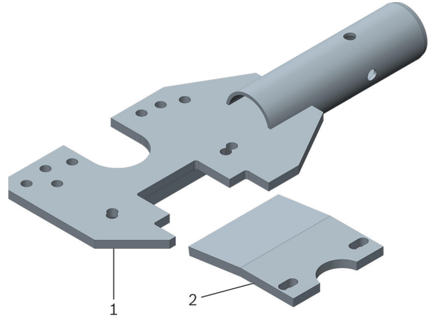
Şekil 1: Dişli kutusu desteği 3221B
