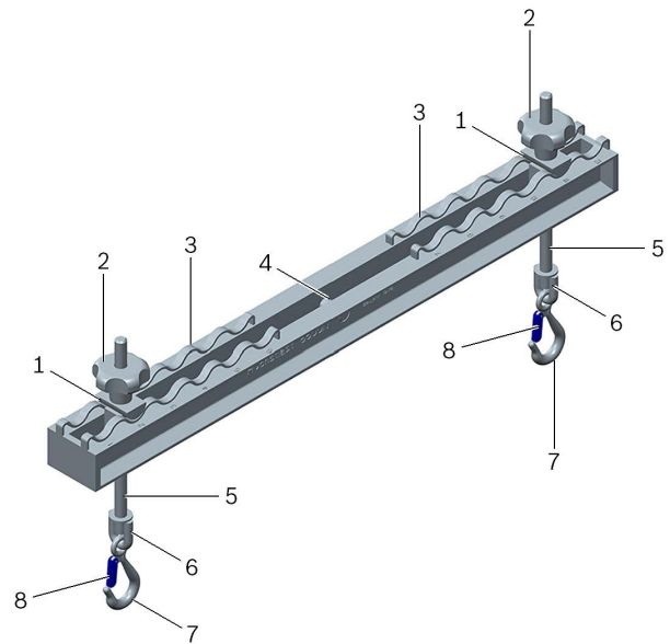
Fig. 1: Attrezzatura di sollevamento 3033
